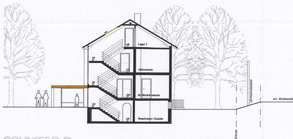
SCHNITT B-B
