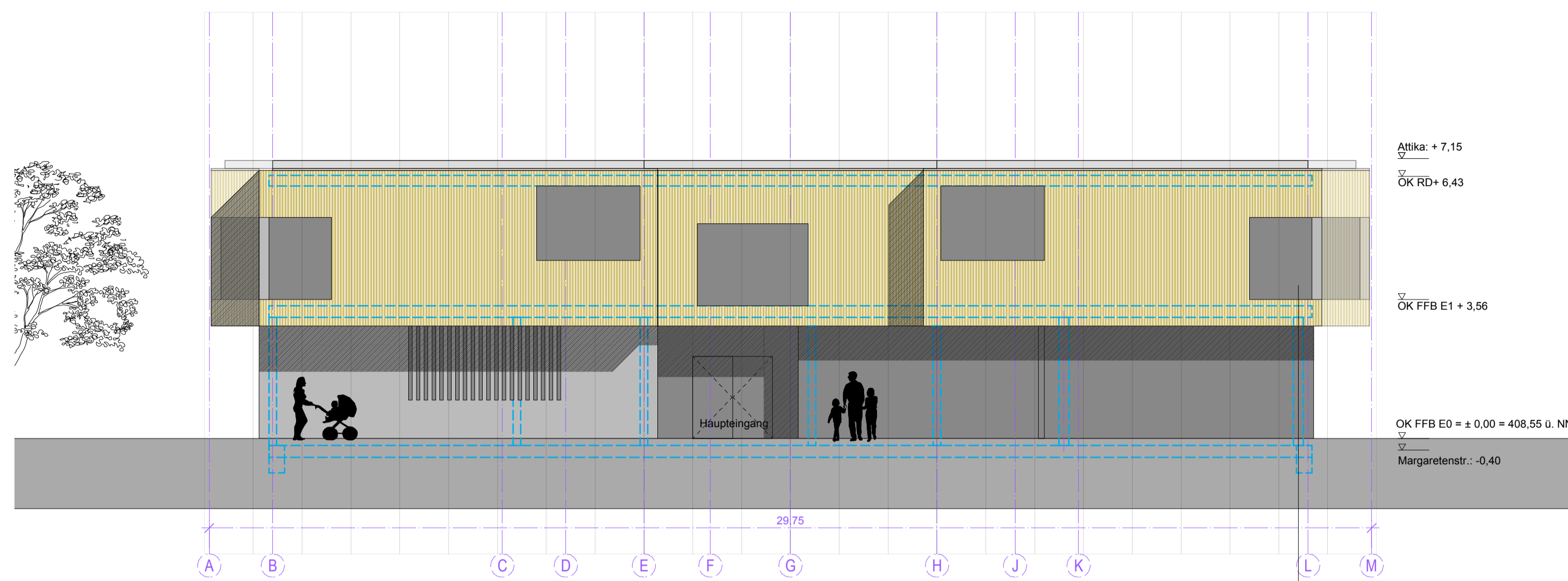
ANSICHT SÜDEN
