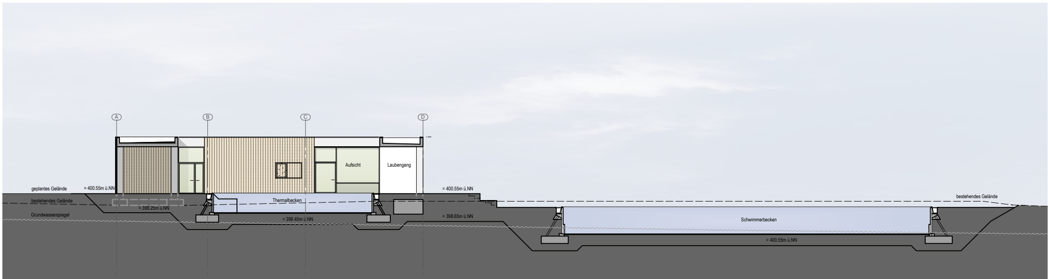
Schnitt A-A
