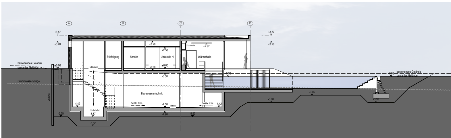
Schnitt B-B
