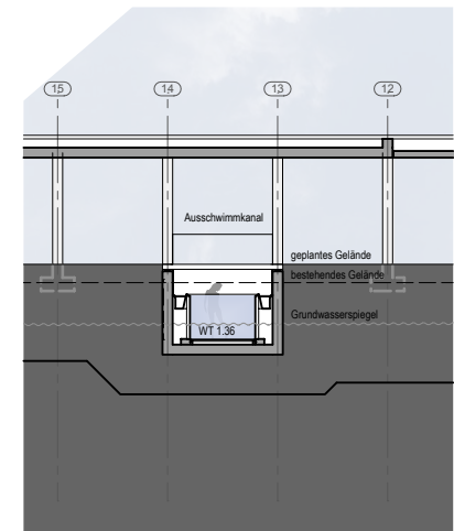
Schnitt O-O
