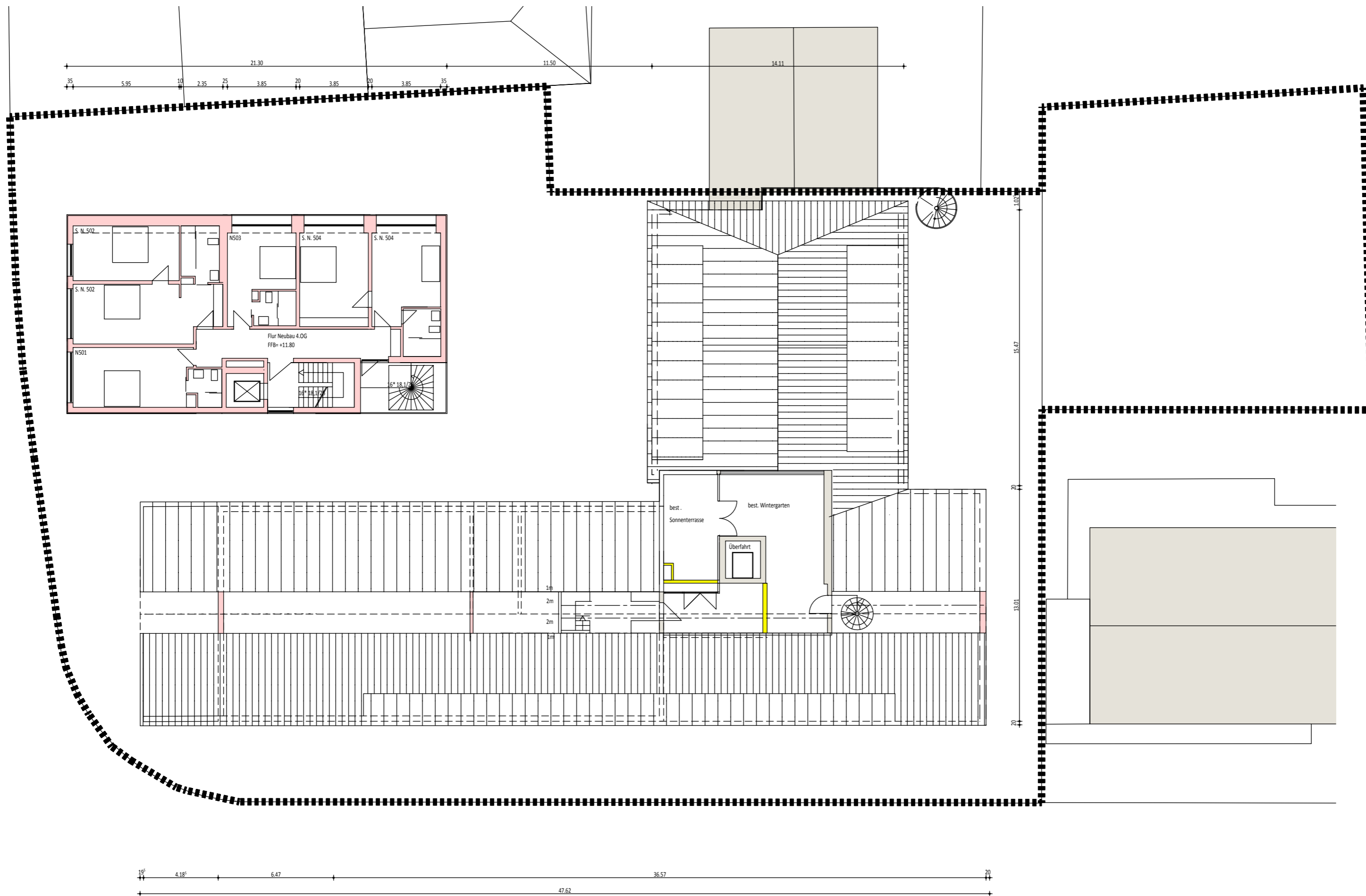
Fennel Hotel Maier - Friedrichshafen - Fischbach Anlage 3: Grundriss 4.OG - 1:200 Entwurf - 05.11.2017
