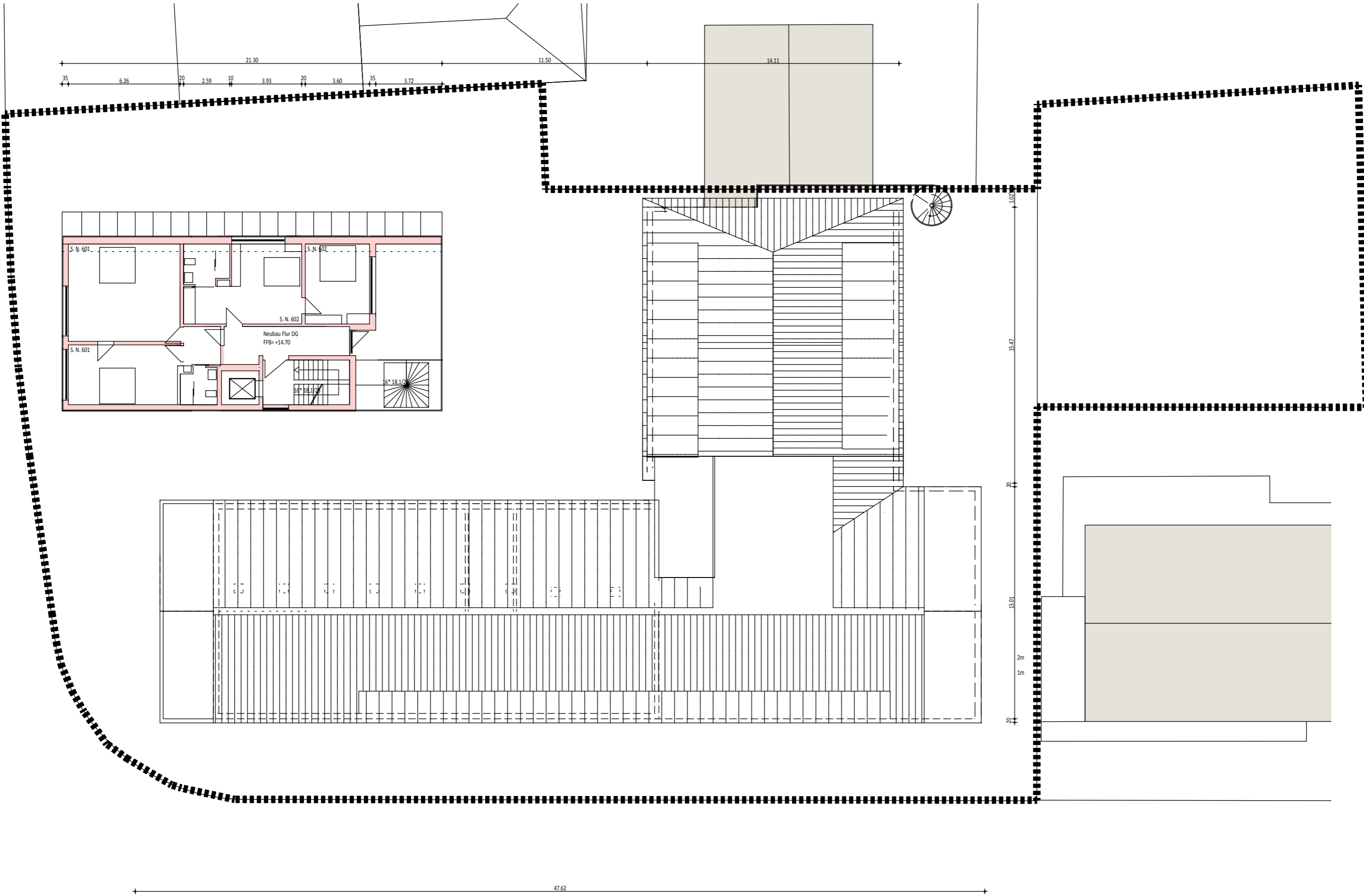
Fennel Hotel Maier - Friedrichshafen - Fischbach Anlage 3: Grundriss DG - 1:200 Entwurf - 05.11.2017
