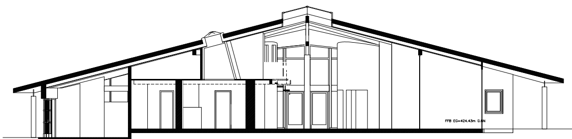
Schnitt A-A
